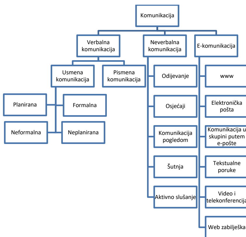
Slika 2. Vrste komunikacije (2)
