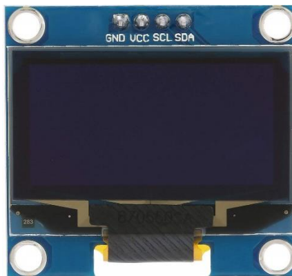
Slika 2.35: 1.3“ OLED displej
