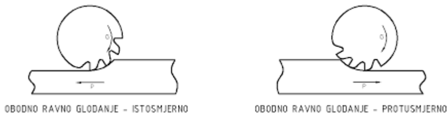
Slika 3.4.1.1 – Kinematike glodanja
