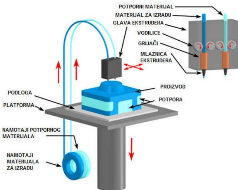
Slika 2.5.1.1 – FDM postupak
