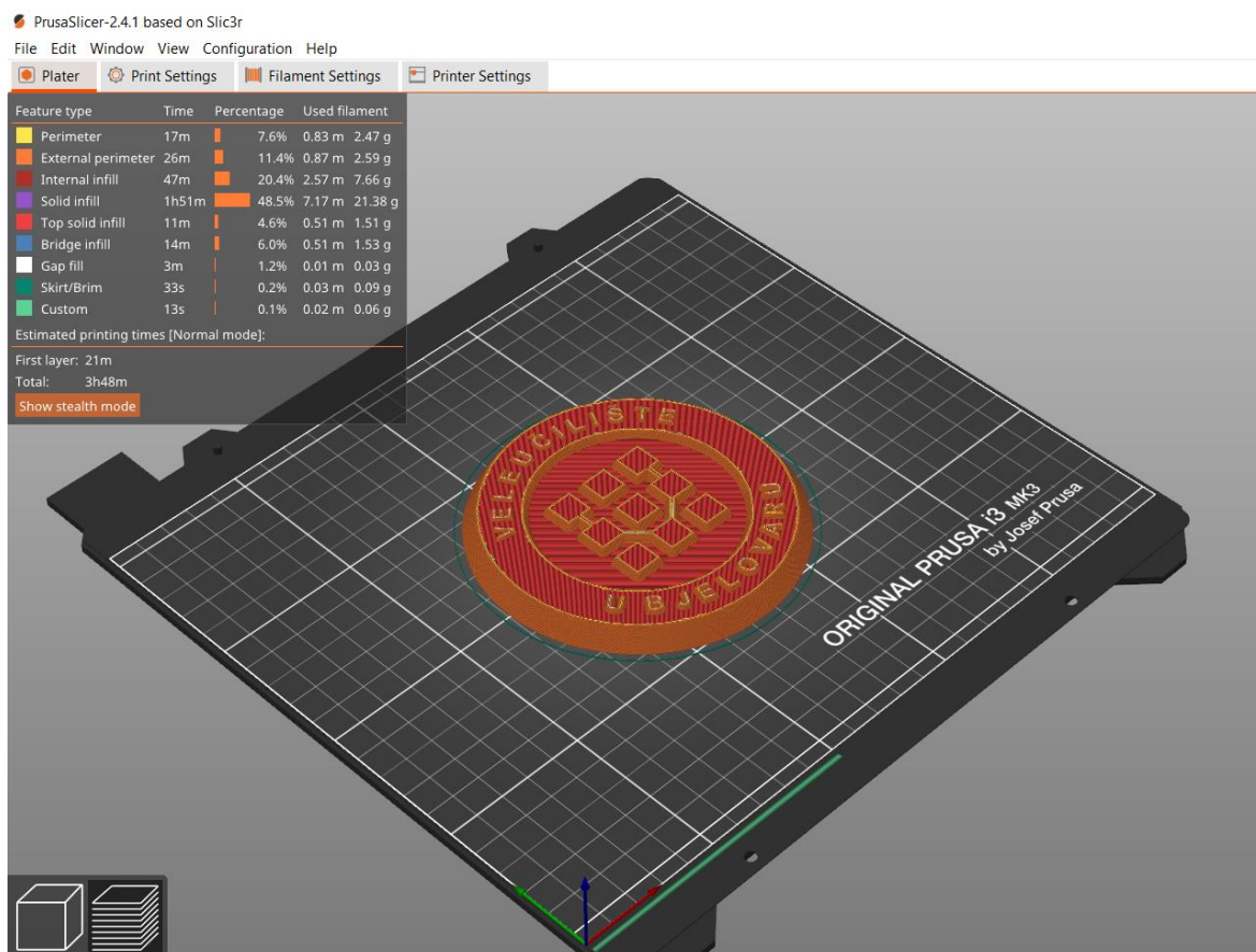
Slika 4.3.2.3 – Prusa Slicer 2.4.1
