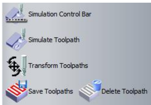
Slika 4.4.2.3 – Naredbe simuliranja
