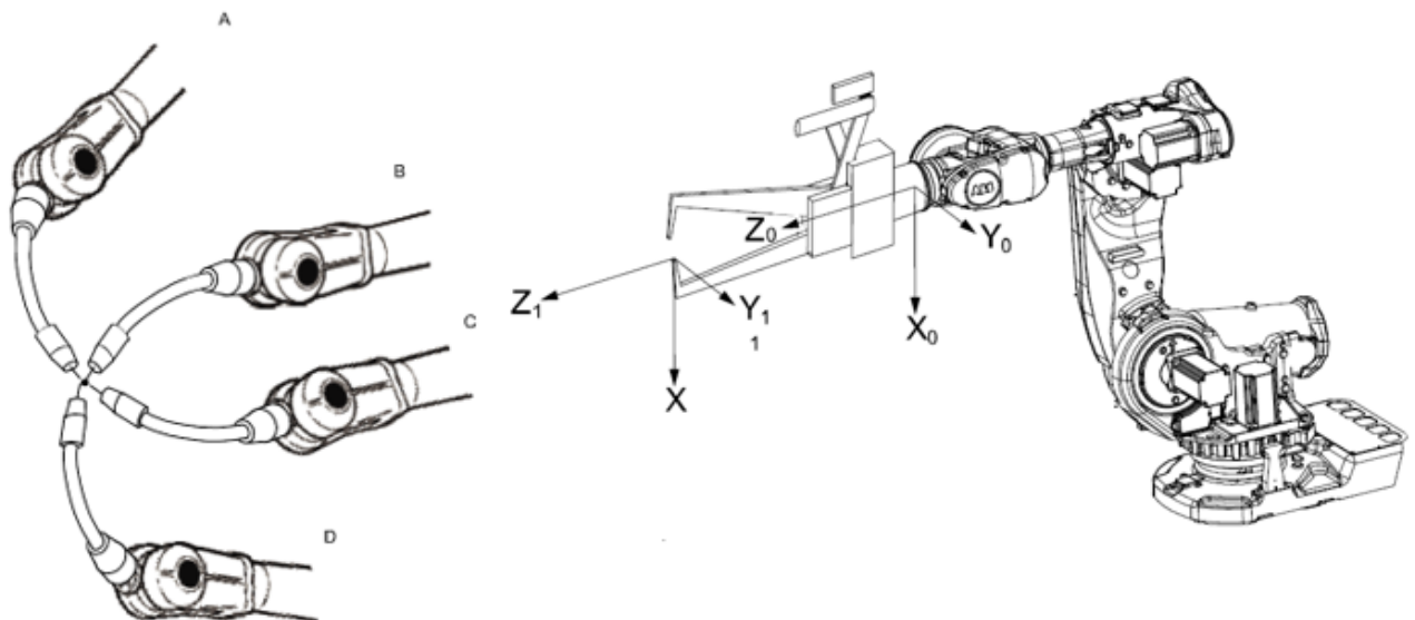
Slika 2.29. Prikaz definiranja TCP-a
