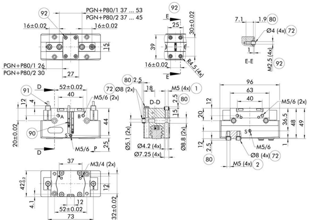
Slika 4.5. Dimenzije prihvatnice s detaljima za montažu [16]
