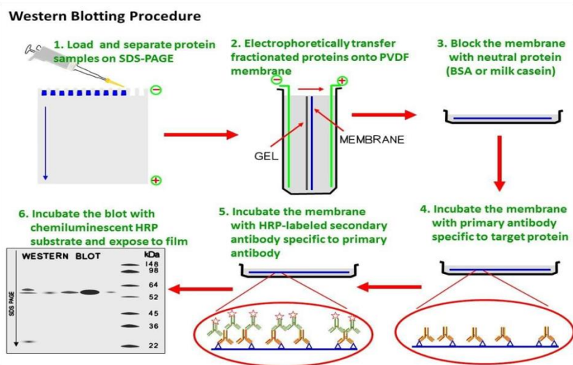
Slika 2.6.1. Western Blotting.
