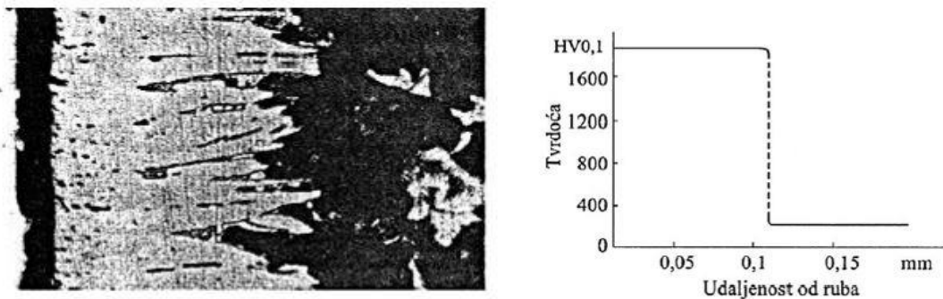
Slika 5.10: Mikrostruktura i prikaz ovisnosti tvrdoće poprečnog presjeka boriranog čeličnog predmeta o udaljenosti od ruba [7]
