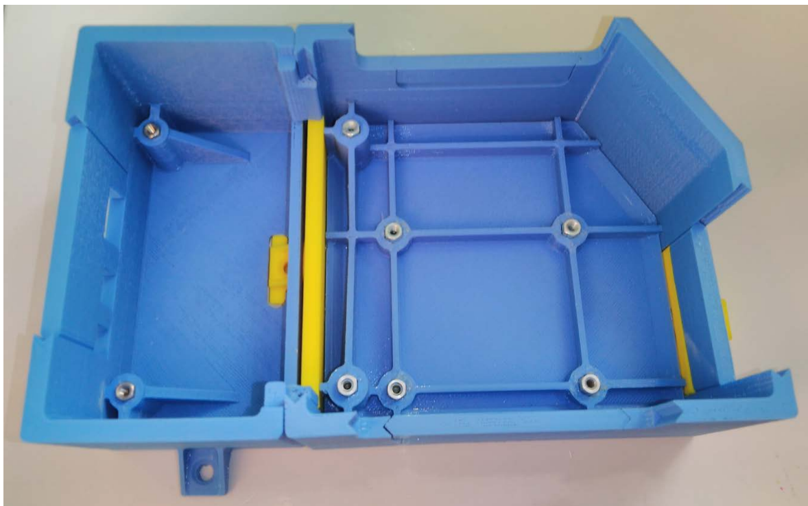
Slika 6.13 Kompletno kućište izrađeno 3D printanjem
