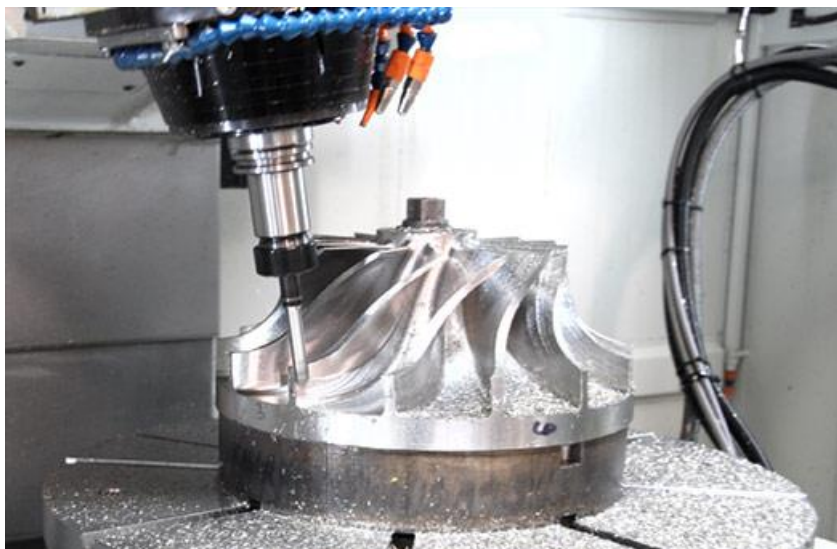
Slika 3.3. Primjer simultanog 5-osnog glodanja [20]
