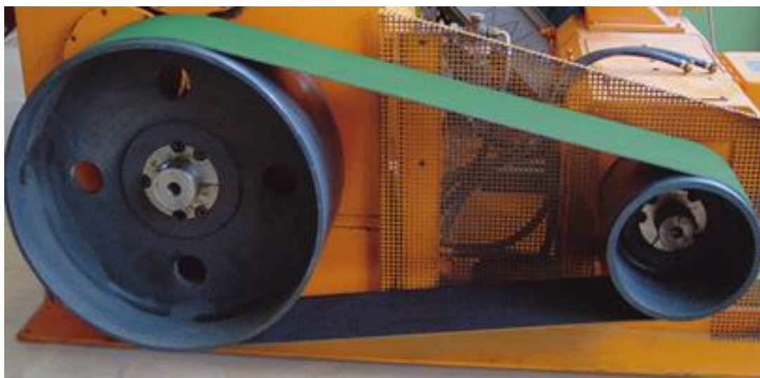
Slika 2.4 Primjer korištenja plosnatog remena [6].
