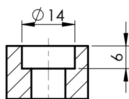
PRESJEK B-B
