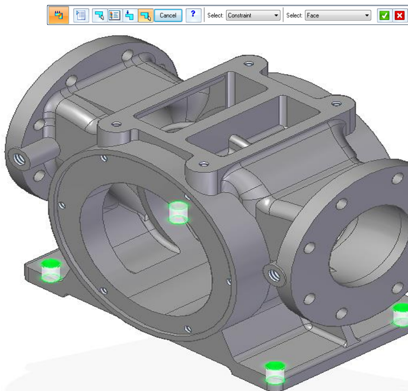
Slika 8.7. Odabir fiksnih oslonaca na kućištu krilne pumpe u programskom alatu SolidEdge ST8
