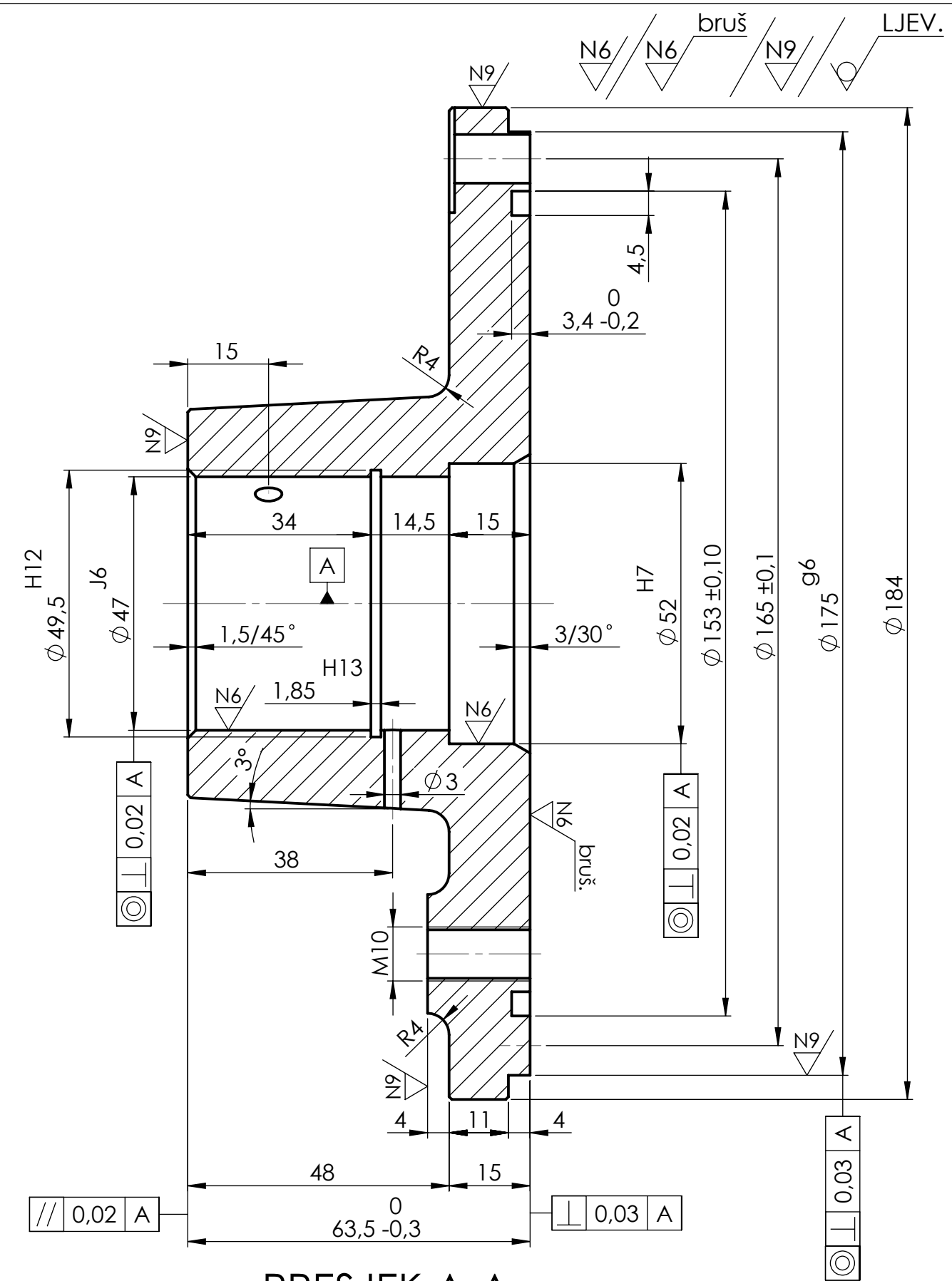
PRESJEK A-A
