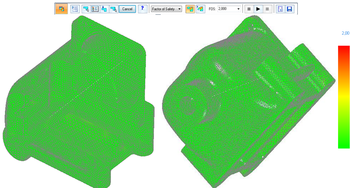
Slika 8.24. Faktor sigurnosti kućišta ventila krilne pumpe za ispitni tlak 1 MPa (10 bar-a) i materijal kućišta SL - 25 (GJL - 250) (FOS – SolidEdge Simulation Express)
