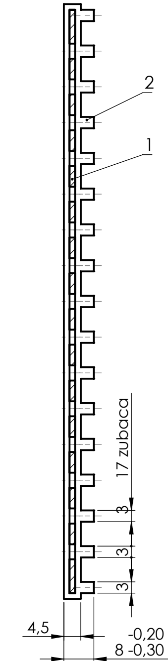
PRESJEK A - A
