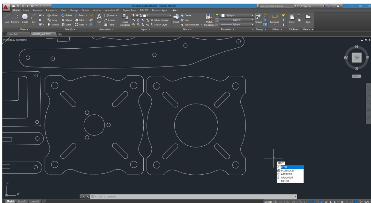
Slika 6.14. Naredba „ PEDIT “
