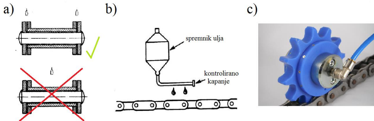
Slika 5.14. Podmazivanje kapanjem, a) isparavan i neispravan način podmazivanja zgloba lanca; b) podmazivanje kapanjem iz spremnika s uljem, c) podmazivanje specijalnim lančanikom [5, 36, 38]
