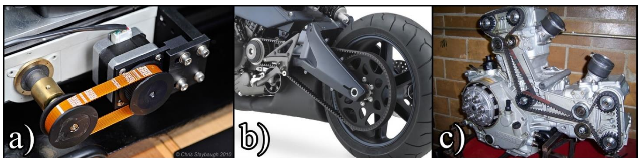
Slika 4.15. Primjeri korištenja zupčastog remena, a) prijenos vrtnje sa step motora; b) završni prijenos motocikala c) razvod bregastih vratila kod Ducati motocikala. [25, 26, 27]
