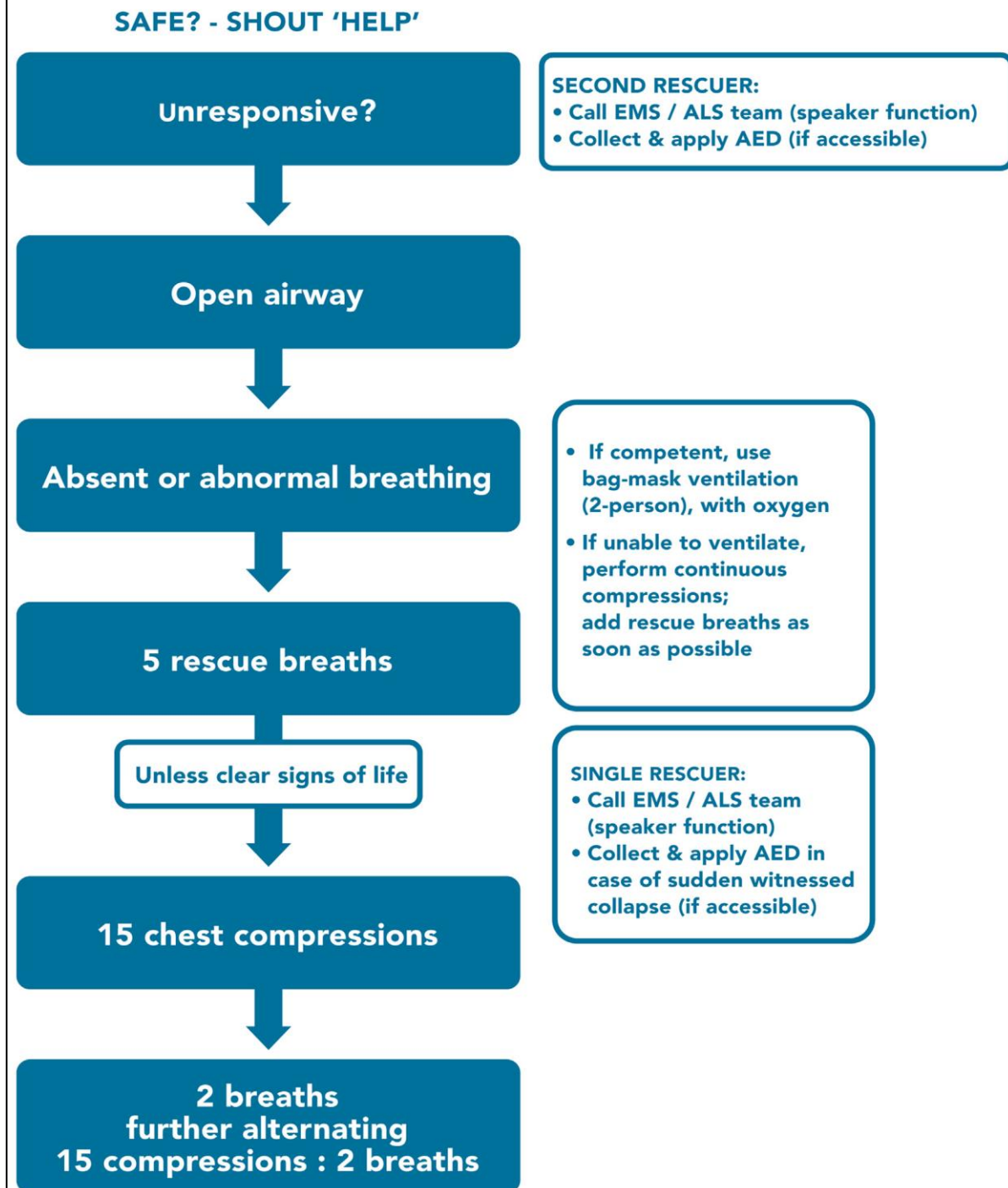
Slika 3.2. PBLS algoritam
