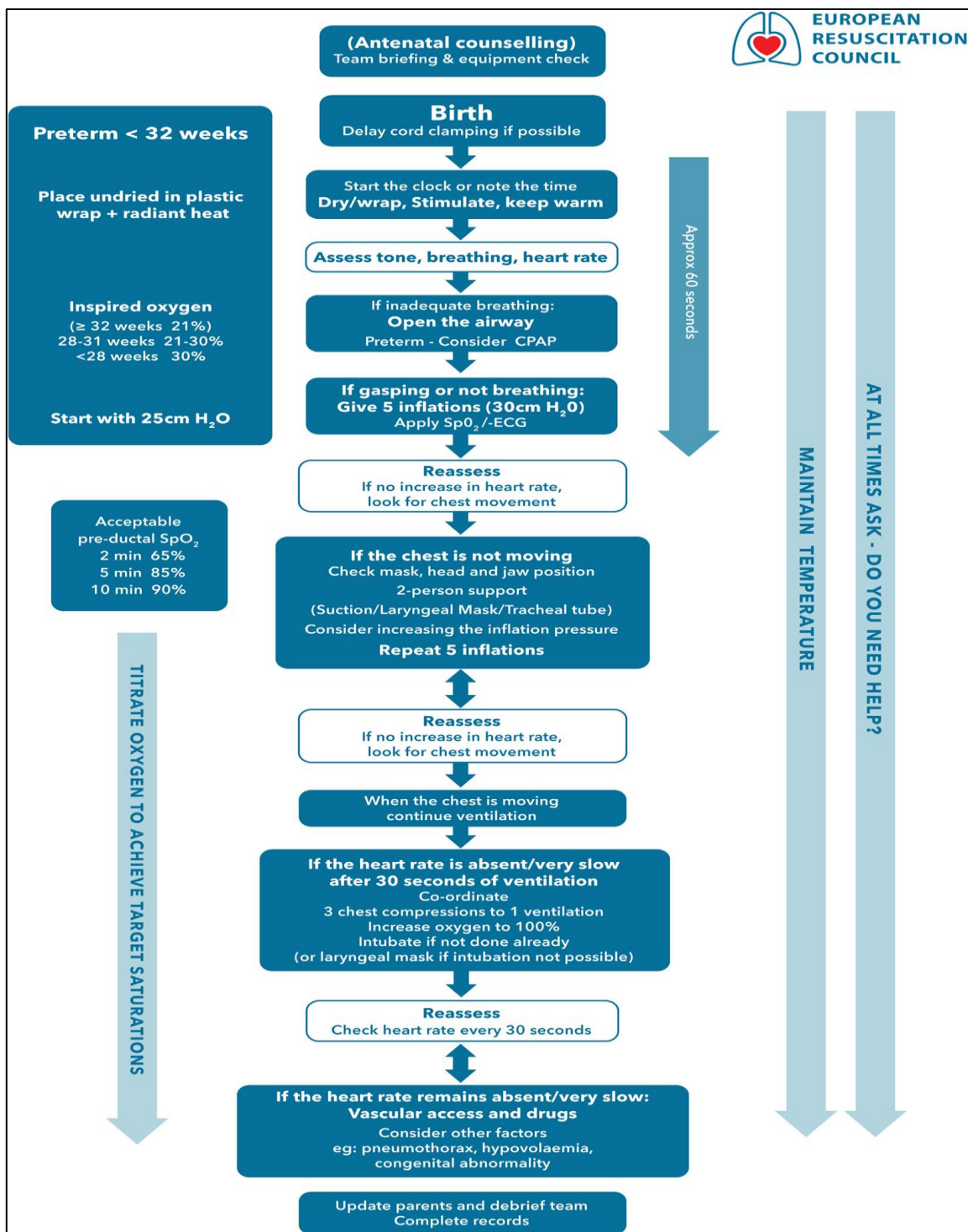
Slika 3.4. NLS algoritam
