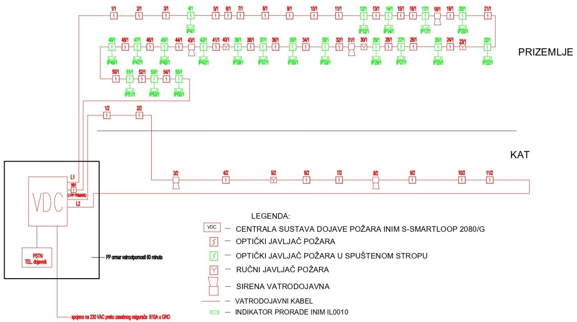
Slika 3.3: Raspored opreme u petlji analogno - adresabilnog sustava vatrodojave [1]
