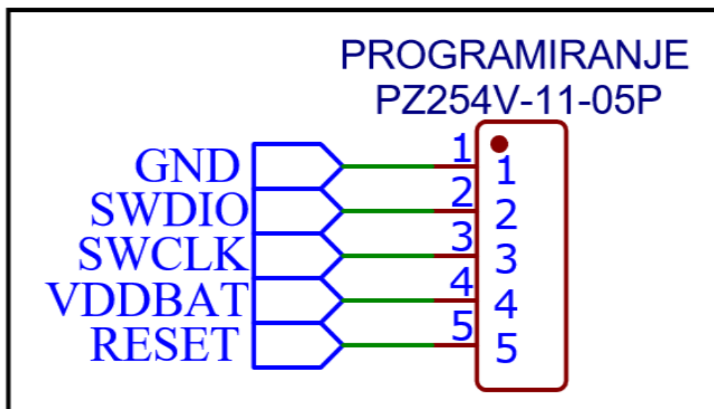
Slika 2.13: Blok programiranje s odgovarajućim konektorom
