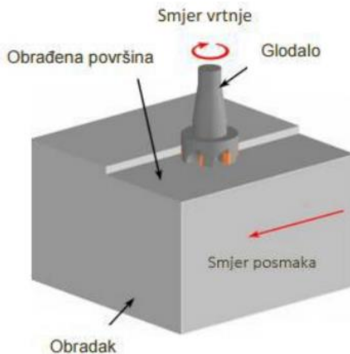
Slika 3.4.1 – Shema glodanja
