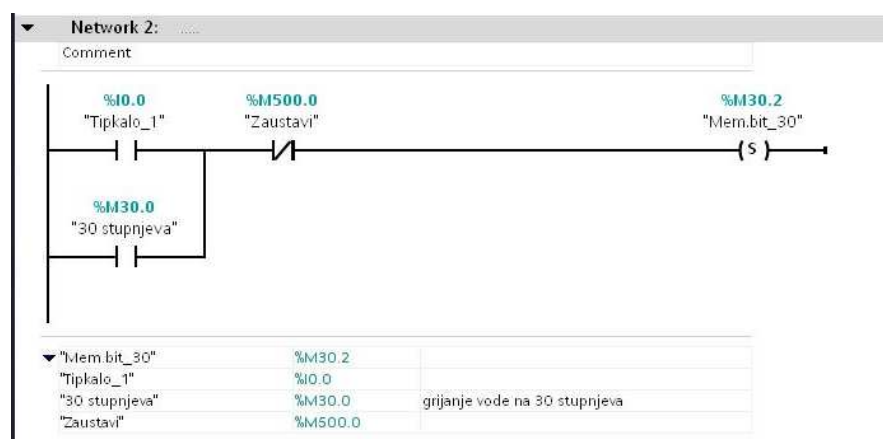
Slika 6.4: Detektiranje aktivacije tipkala 30 stupnjeva
