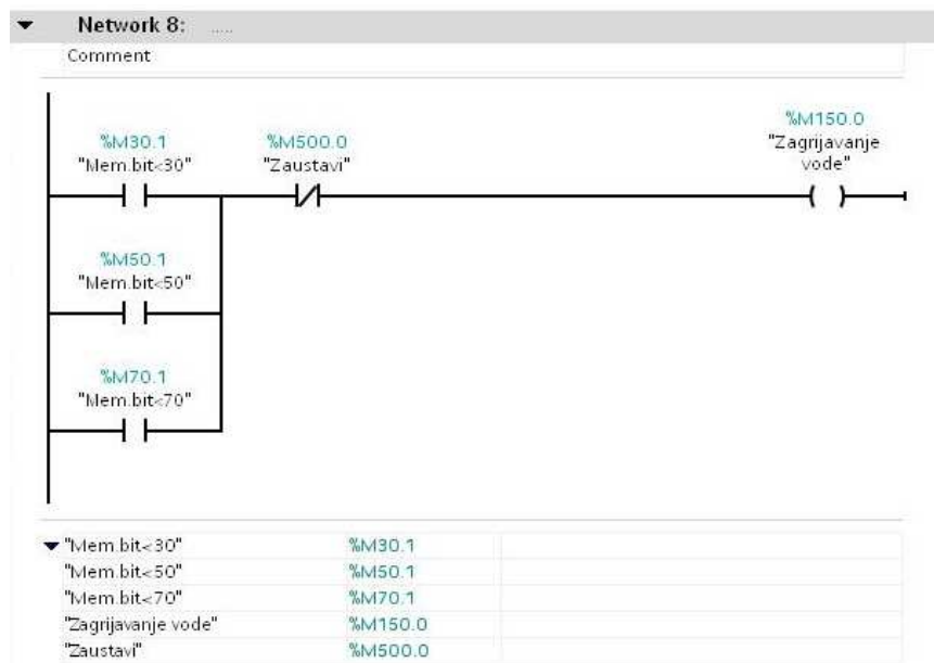
Slika 6.10: Aktivacija memorijskog bita za zagrijavanje vode
