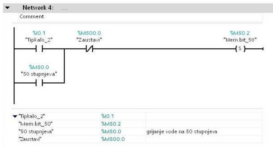
Slika 6.6: Detektiranje aktivacije tipkala 50 stupnjeva
