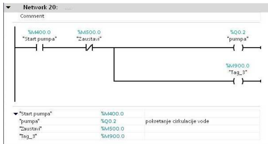
Slika 6.22: Aktivacija izlaza PLC-a „pumpa“
