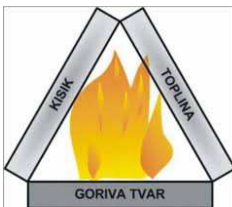
Slika 1.1: Vatrogasni trokut [2]
