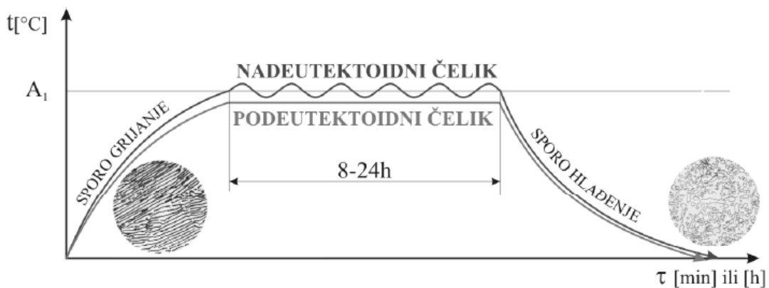
Slika 3.8: Dijagram postupka sferoidizacije [12]
