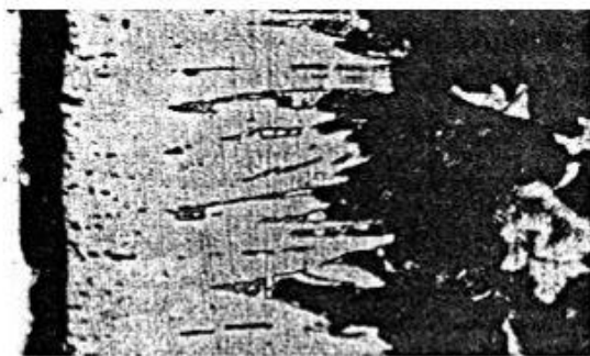
Slika 5.10: Mikrostruktura i prikaz ovisnosti tvrdoće poprečnog presjeka boriranog čeličnog predmeta o udaljenosti od ruba [7]
