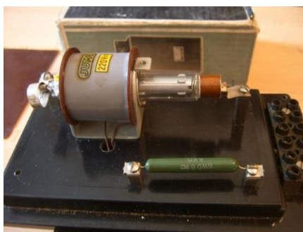
Slika 3.21: Živin prekidač [21]
