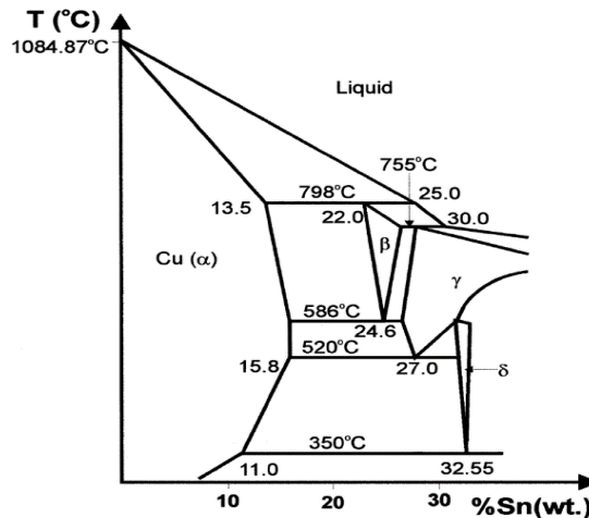
Slika 3.7: Dijagram Cu-Sn [10]
