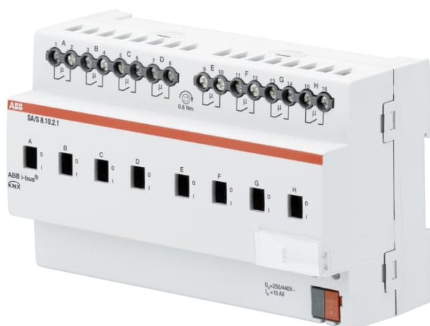
Slika 5.8. ABB SA/S8.10.2.1 KNX relejni aktuator [13]
