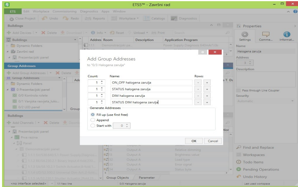
Slika 9.5. Postavljanje grupnih adresa unutar podgrupa
