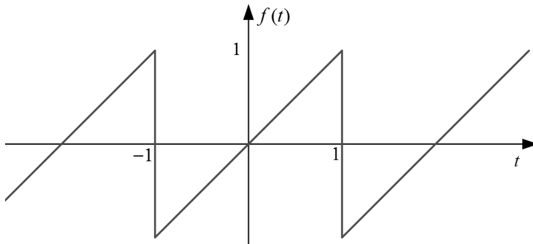
Slika 8.9: Neparna funkcija f(t)
