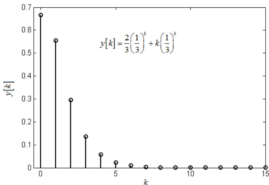
Slika 11.7: Rješenje nehomogene diferencijске једнадџбе y[k] - \frac{1}{3}y[k-1] = \left(\frac{1}{3}\right)^k, k \geq 0 , početni uvjet: y[-1] = -1 .
