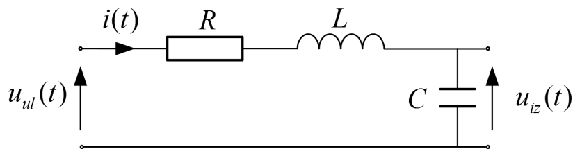
Slika 4.11: RLC krug
