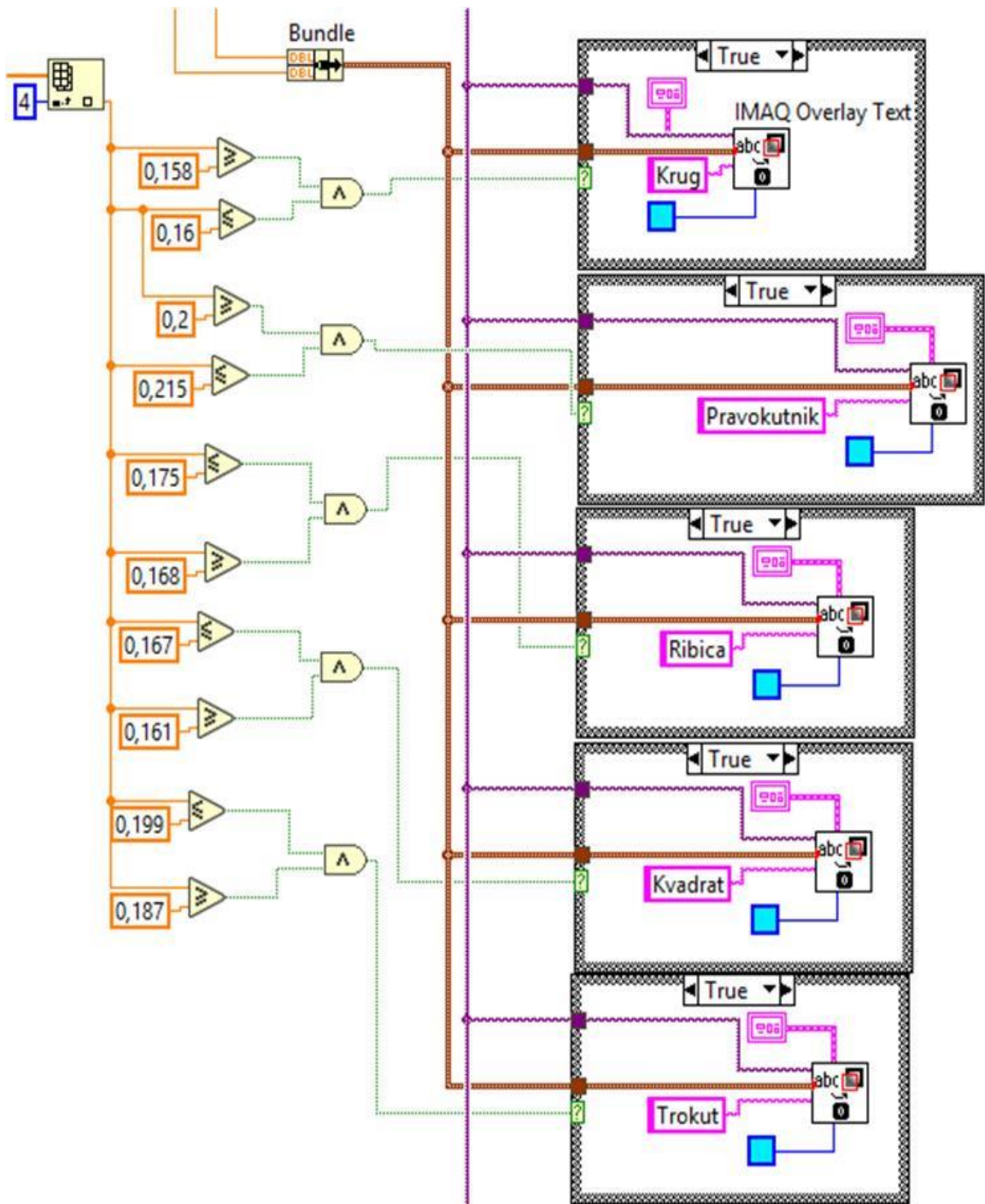
Slika 7.5: Klasifikacija objekata
