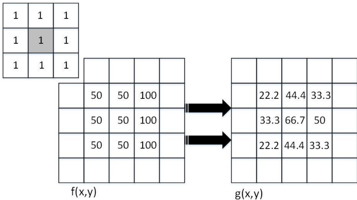
Slika 6.5: Princip rada prostornog filtera
