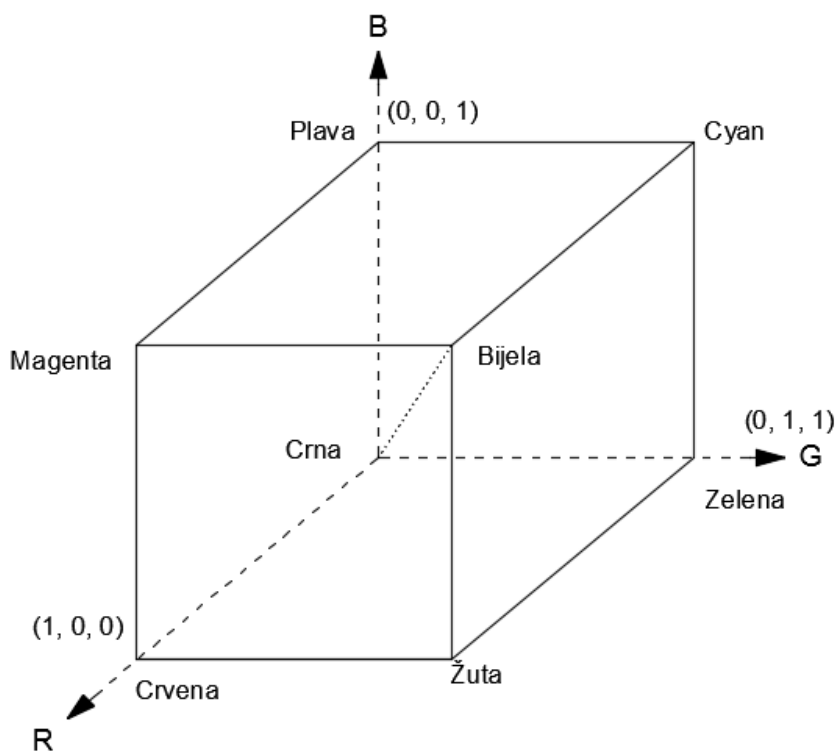
Slika 6.2: RGB sustav [10]
