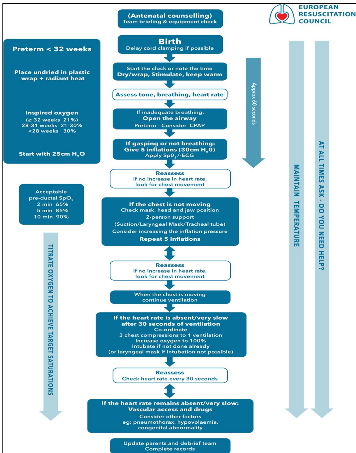
Slika 3.4. NLS algoritam
